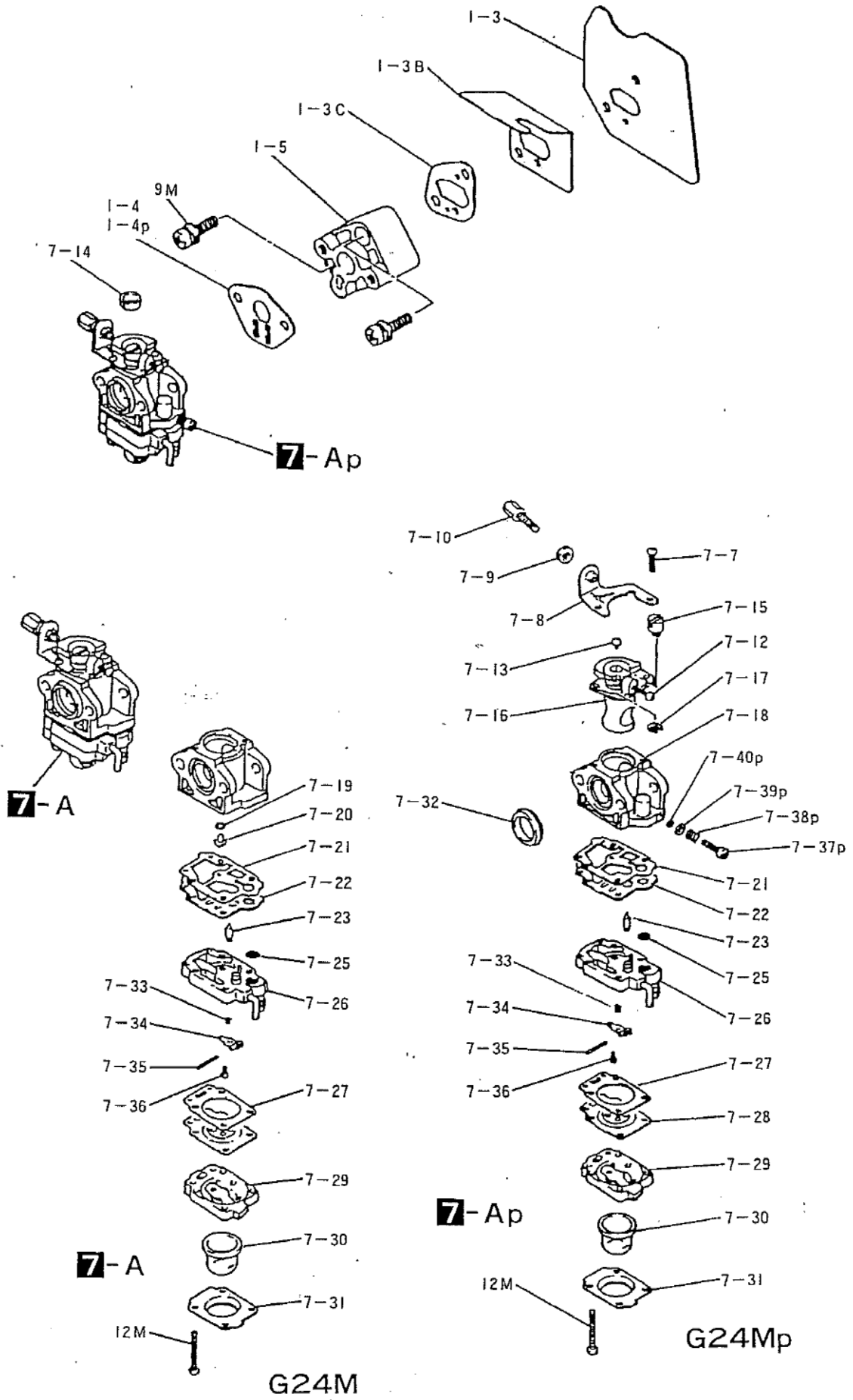
G24M/p 新キャブレタ部品
